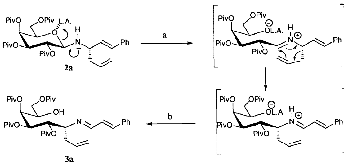
Scheme 2: a: Lewis acid L.A.; b: Hydrolysis.
